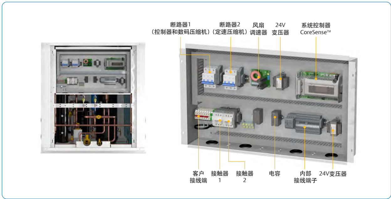
图3. 12-16HP机组的电气模块
