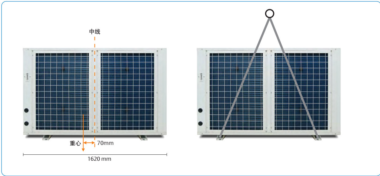
图11. 12-16HP机组吊装图
