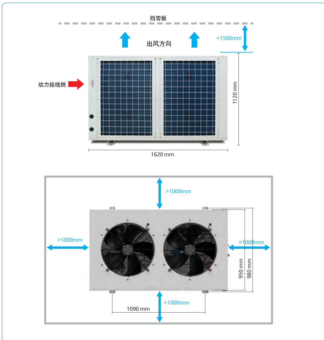
图9. 12-16HP室外型机组外形尺寸
