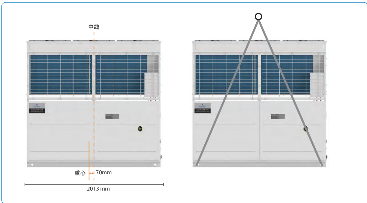
图12. 20HP机组吊装图
