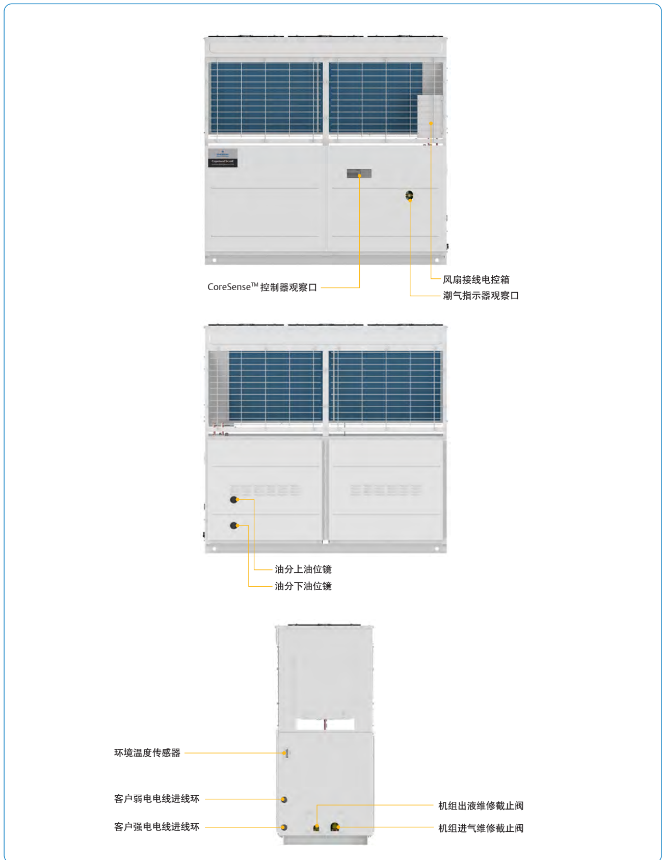
图5. 20HP机组外形
