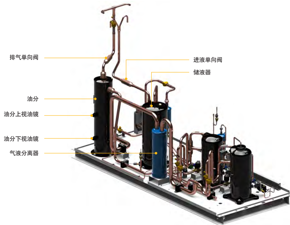
图6. 20HP机组的主要部件
