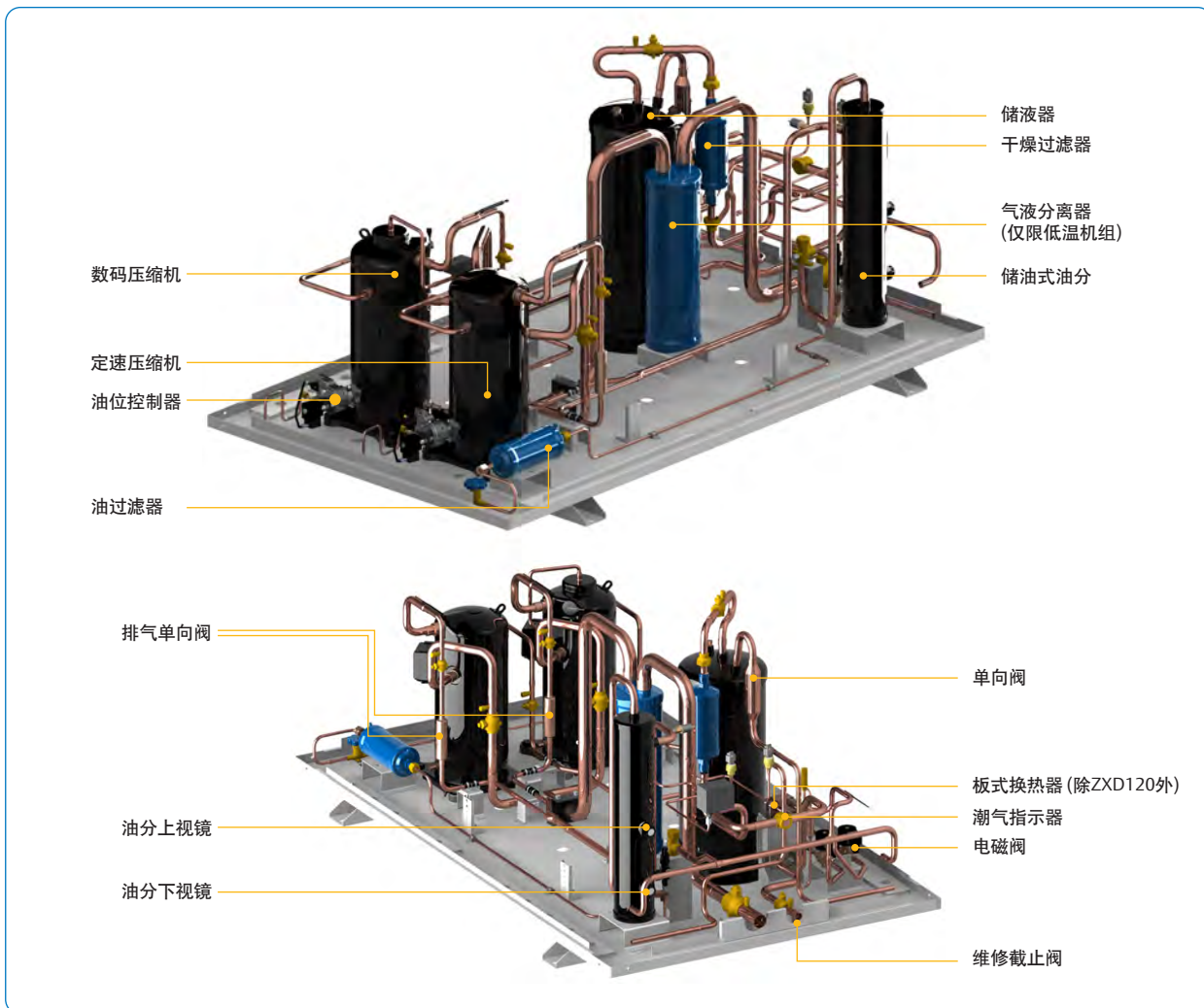
图2. 12-16HP机组的主要部件
