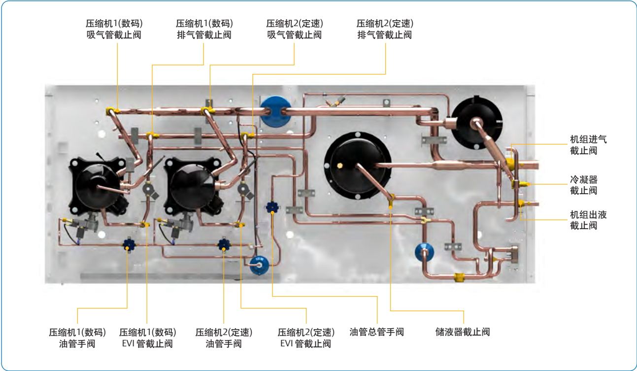
图8. 20HP机组的维修服务阀
