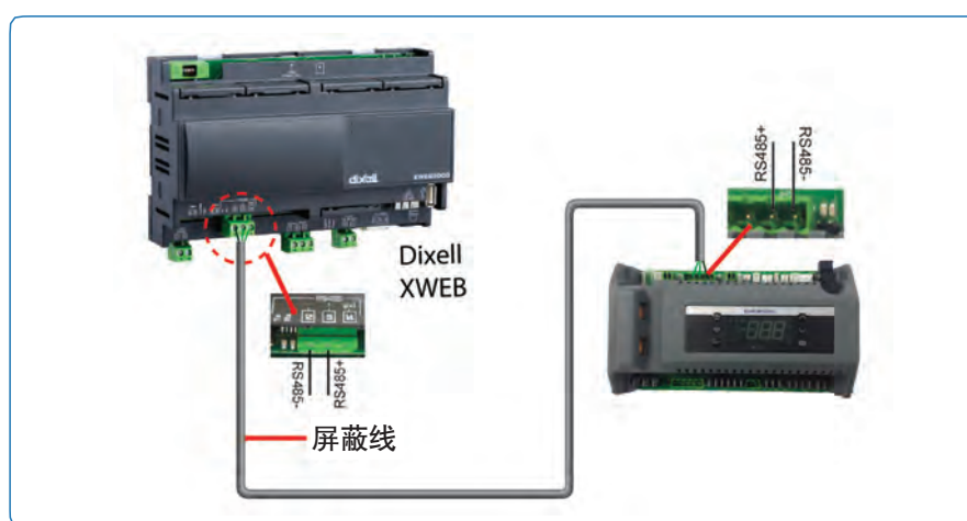
XWEB与智能店解决方案模块接线
