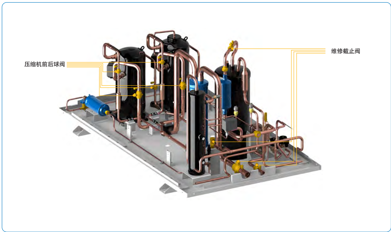
图4. 12-16HP机组的维修截止阀
